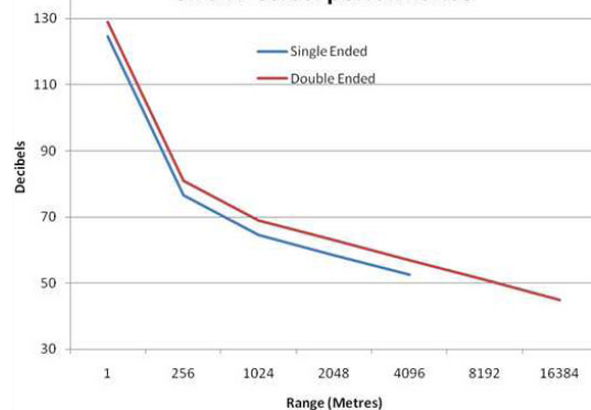
Siren Decibel performance
